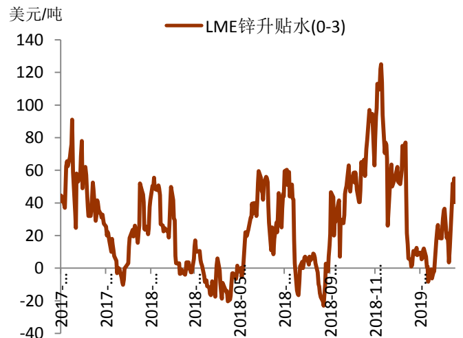
图 4 LME 升贴水
